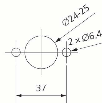
vrtání otvorů pro magnetické rozety
