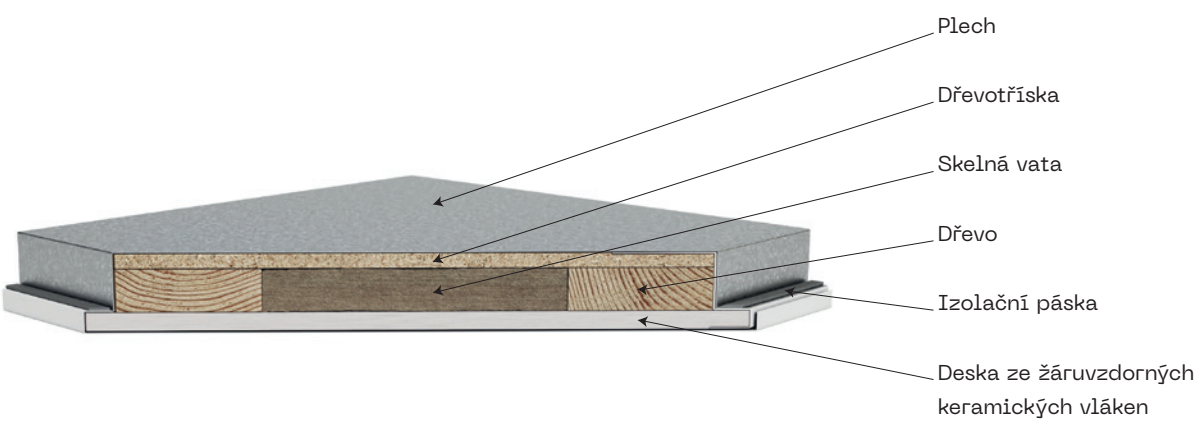
PROTIPOŽÁRNÍ SCHODY: ŘEZ DOLNÍM VÍKEM
