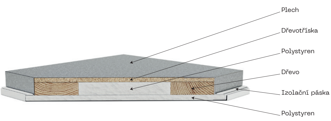
ZATEPLENÉ SCHODY: ŘEZ DOLNÍM VÍKEM
